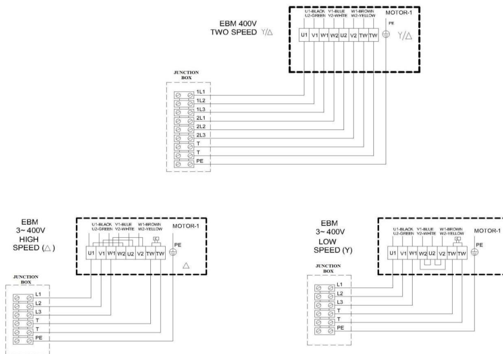
Figure 7. Schéma de raccordement ventilateur 400V (EBM)
