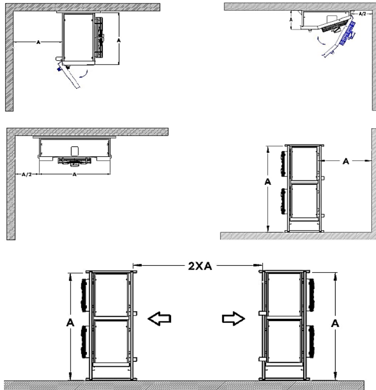
Figure 4. Positionnement des refroidisseurs à l'intérieur de la chambre
