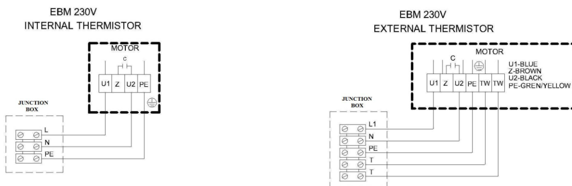
Figure 5. Schéma de raccordement ventilateur 230V (EBM)
