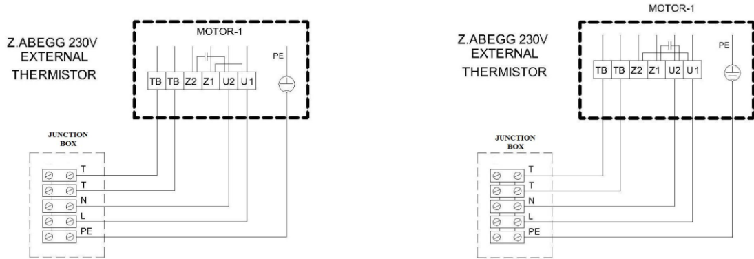
الشكل 6. مخطط توصيل مروحة 230 فولت (Z.ABEGG)
