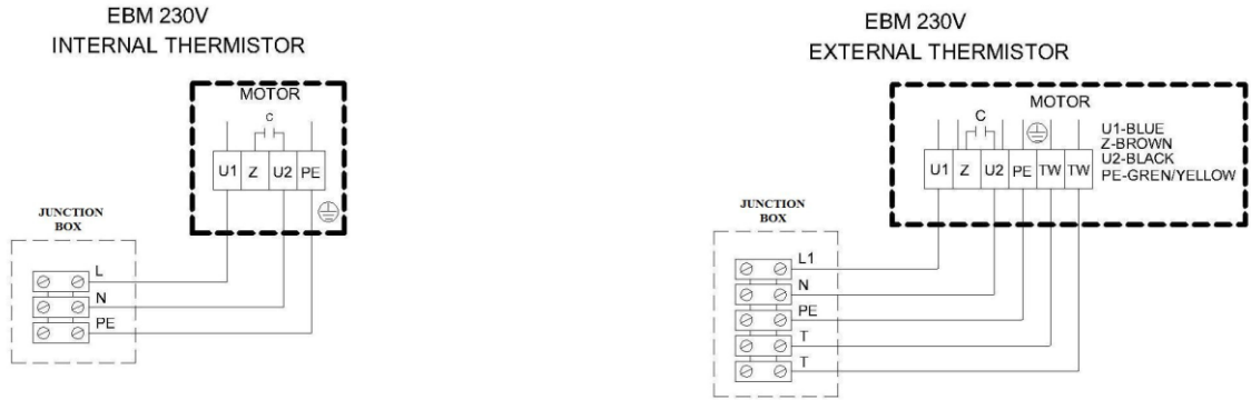
الشكل 5. مخطط توصيل مروحة 230 فولت (EBM)
