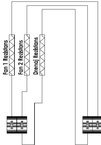
الشكل 11. مخطط توصيل المروحة والسخان وتصريف المياه
