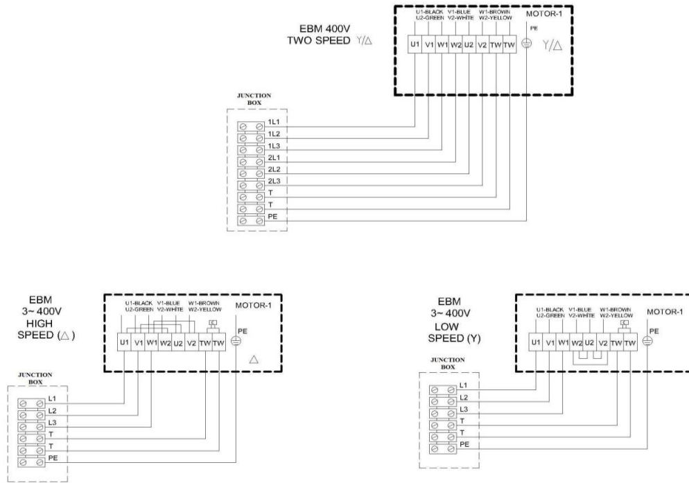
الشكل 7. مخطط توصيل مروحة 400 فولت (EBM)
