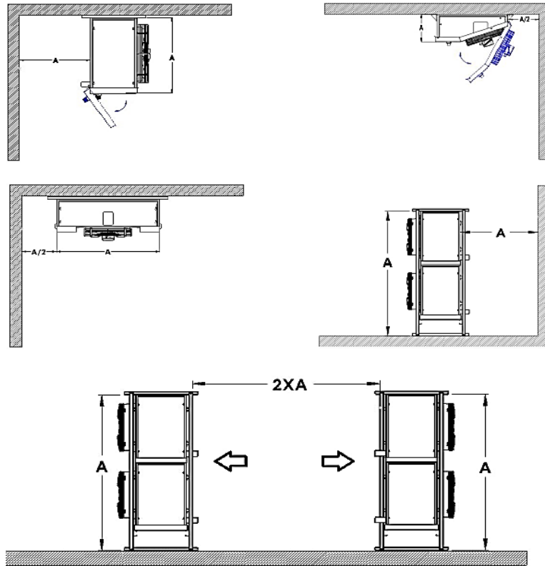
الشكل 4. تمركز المبردات داخل الغرفة
